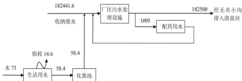
图 2-1 项目水平衡图
